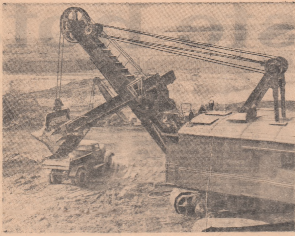
Cupa uriașă a excavatorului dislocă încă un strat de steril, pentru a ajunge la cărbune. În acest fel, se pregătește un nou front de lucru la situl Exploatarea minieră Rovinari
