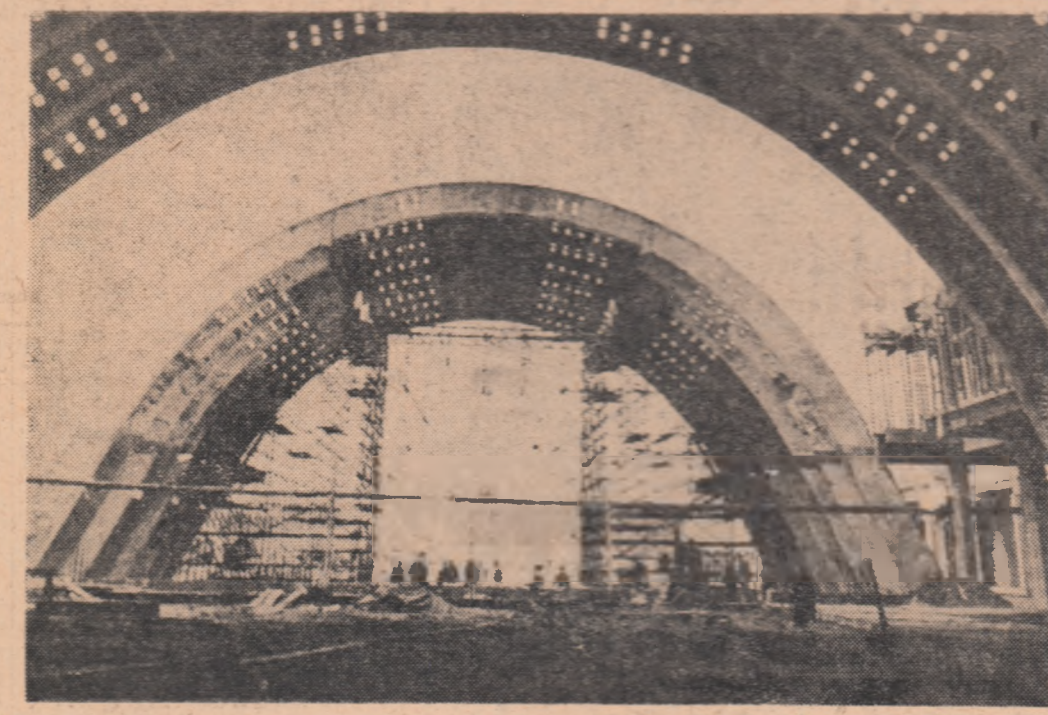
R.P. POLONA: aspect de pe șantierul de construcție al unui depozit de produse linate la uzinele de nitrogen din Polonia
