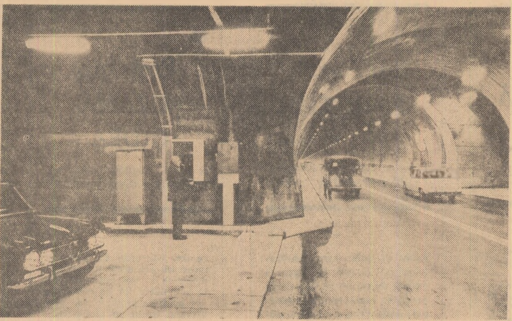
Agencia France Presse anunță că tunelul săpat pe sub Mont Blanc între Franța și Italia va fi inaugurat la 16 iulie. Tunelul are o lungime de 12 km și a fost săpat la cotele 1200-1300 m. El va putea fi utilizat și iarna, chiar atunci cînd ninge abundent. Se prevede că pe această autostradă vor circula 400.000 de autovehicule anual, adică aproximativ 1.500 pe zi. O jumătate din lucrare a fost realizată de Italia, iar cealaltă de o societate franceză. În fotografie: vedere parțială a tunelului
