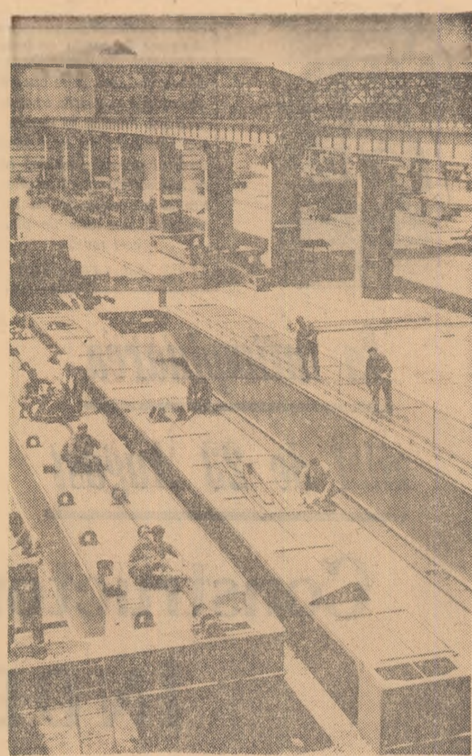
Uzina de construcții metalice și mașini agricole Bocsa. Se montează un nou pod rulant de 12,5 tone pentru halele industriale
