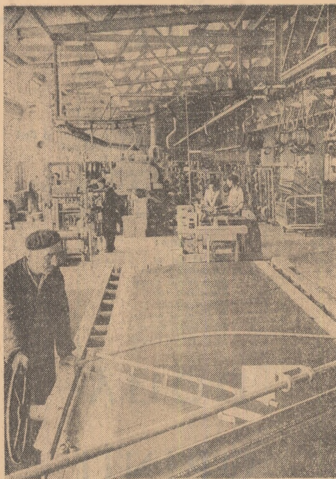
Uzina „Victoria”-Florești, regiunea Ploiești, și-a îndeplinit angajamentele luate în cinstea zilei de 23 August. Aspect din noua hală de producție a garniturilor auto moto, velo a uzinei
