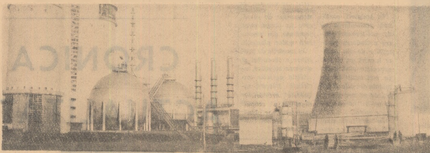
Vedere generală a Combinatului de Îngrășăminte azotoase din orașul Tg. Mureș Foto: AGERPRES
