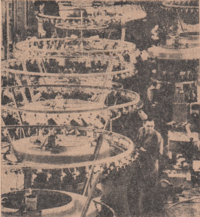
R. D. GERMANĂ. — Noi mașini moderne de tricout în curs de montare la fabrica de tricotaie Mitweide
