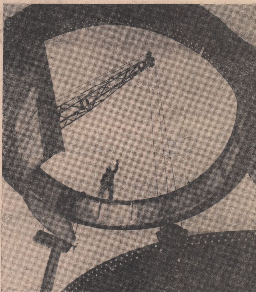
Pe azurul cerului glădețean se profilează imense rotunde metalice. O comandă precisă și urlașul de oțel se supune docil voinței montorilor unui nou obiectiv din zona sudică a Combinatului siderurgic din Galați
