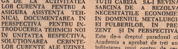
Elevii al Grupului școlar al U.C.R.C.O.M. din Focșești lucrează, sub îndrumarea mîntorului, la remedierea unor defecte ale televizorului
