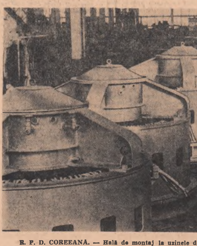
R. P. D. COREEANA. — Hală de montaj la uzinele de mașini electrice din Daian
