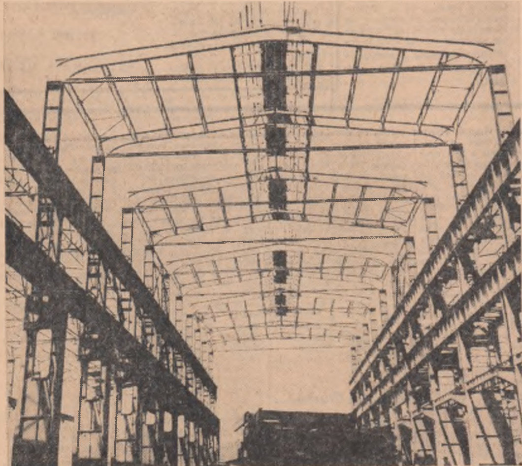
Uzina metalurgică Bucureşti. Vedere parţială a noii hale de turnătorie aflată în construcţie. Foto: AGERPRES
