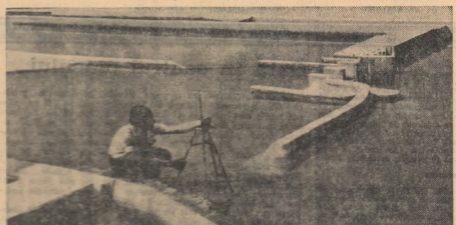
Instalația de studii și cercetări hidrotehnice din Capitală. Se studiază la scară reală închiderea albiei de la sistemul hidroenergetic și de navigație de la Porțile de Pier, preconizată pentru anul 1980.
