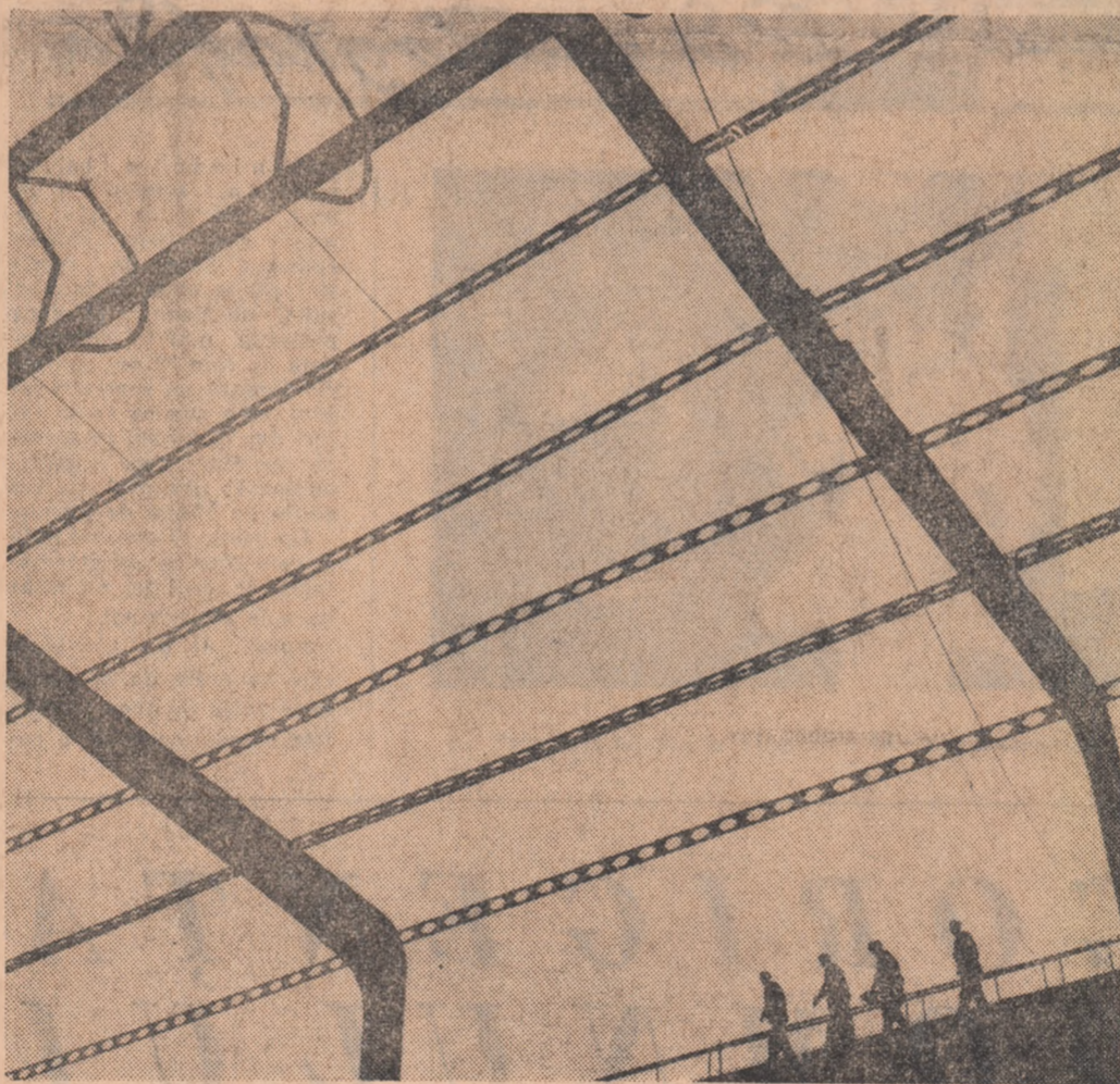
Geometrie dinamică
