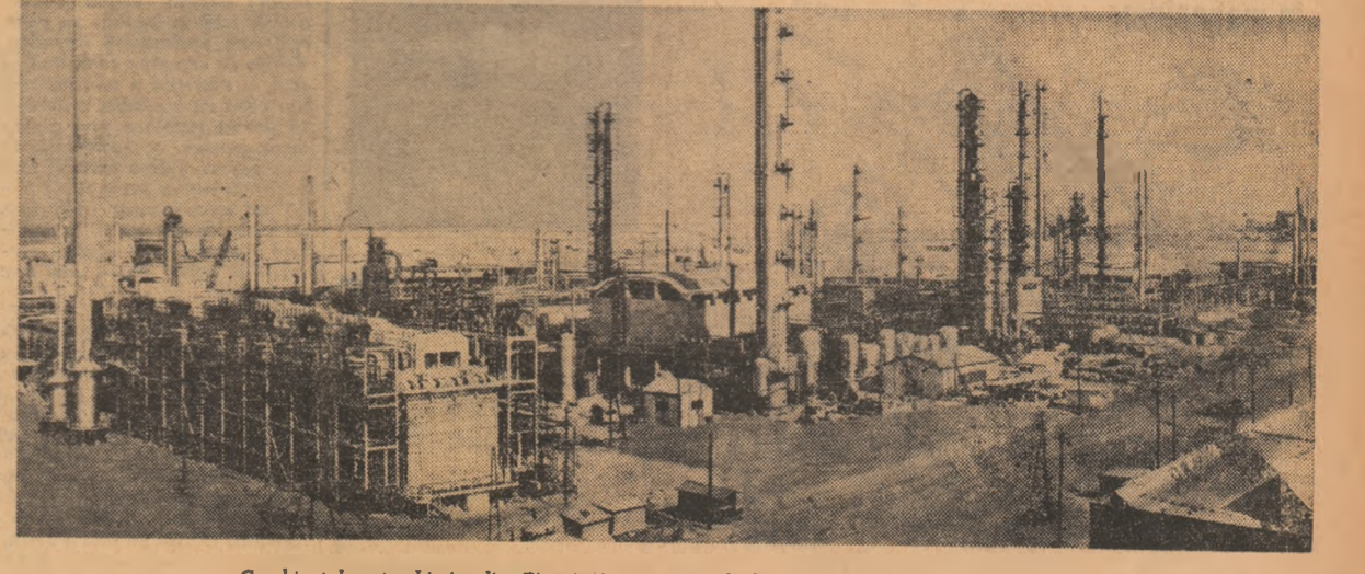
Combinatul petrochimic din Pitești. Aspect general al instalației de piroliză a benzinei
