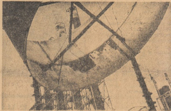
Rafinăria Fitești. Se montează un nou tronson la coloana de fracționare-distilare apă
