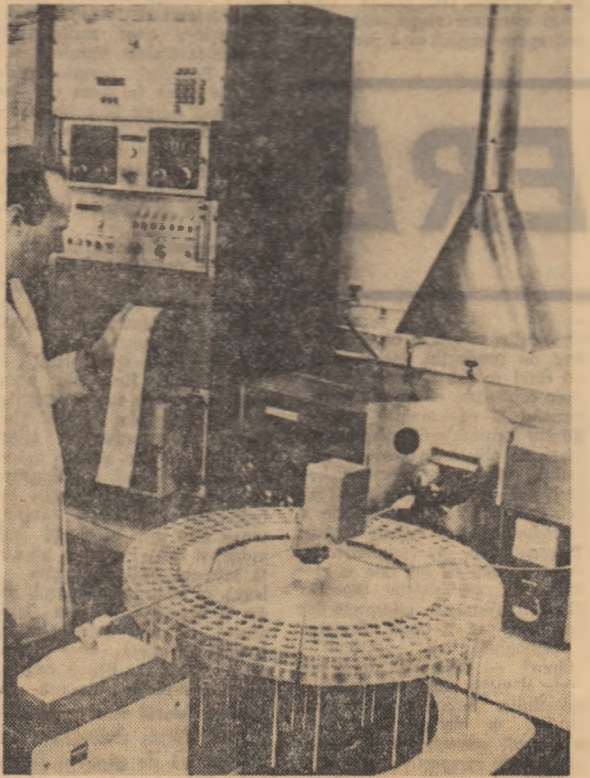
In foto: Sistem automat de absorbție, proiectat de Corporația Perkin-Elmer din Norwalk (Connecticut), destinat analizării conținutului de metale din serul sanguin...
