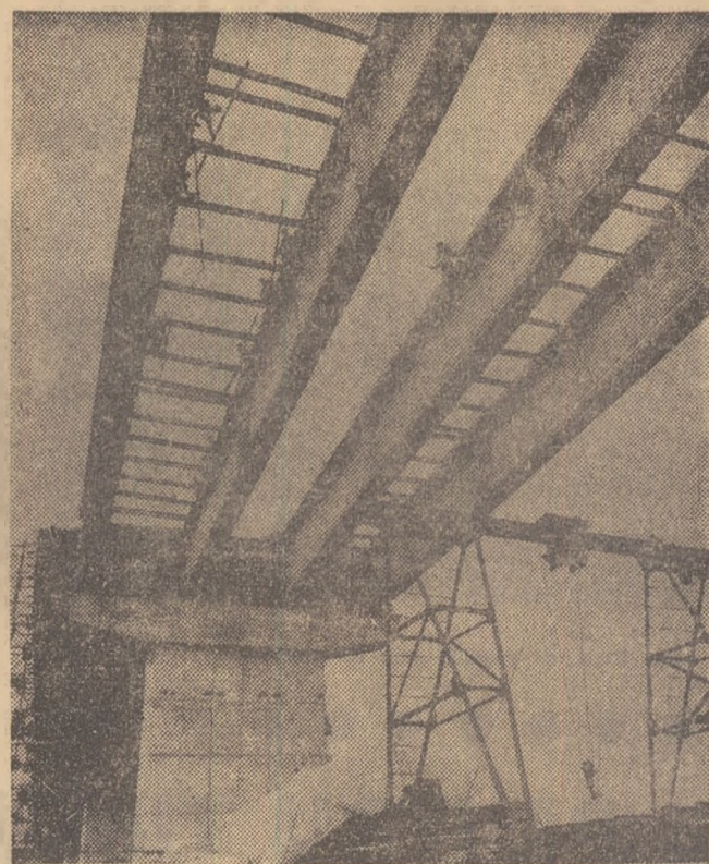
Șantierul pod-Dundre din punctul Giurgeni - Vadul Oii. Brațele harnice ale oamenilor ridică în acest loc unul dintre cele mai mari poduri, creând astfel puntea rutieră între Dobrogea și restul țării
