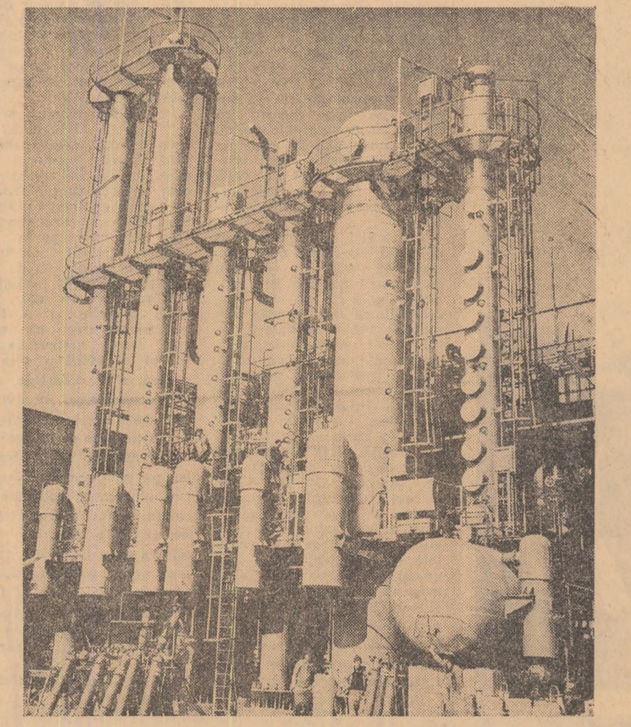
Coloanele de distilare metanol-glicon. (Uzina de fibre sintetice din Iași)
