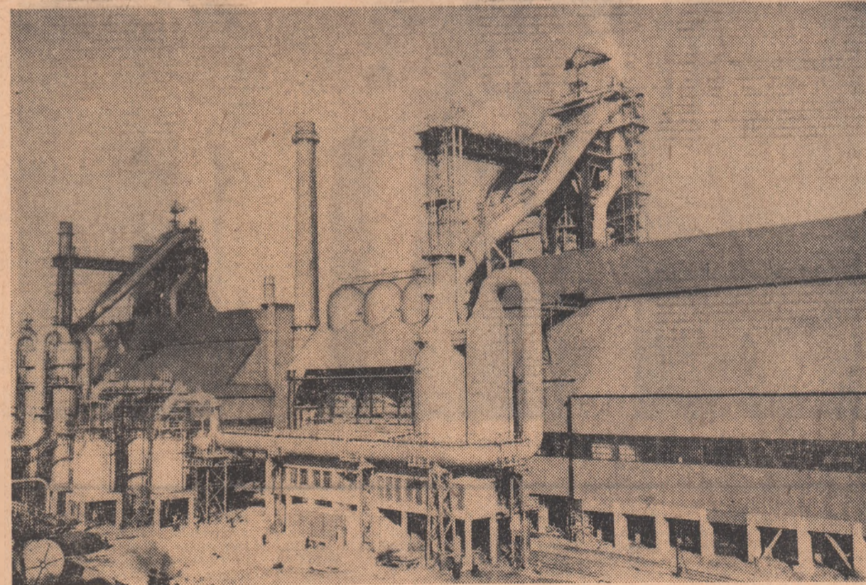
Vedere de ansamblu a celor două furnale de 1700 mc. ale Combinatului siderurgic din Galați.
