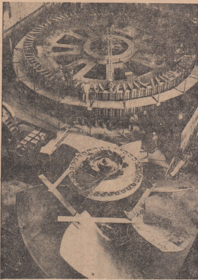
In imagine aspect de la montarea rotorului turbinei nr. 1 și a rotorului generator al aceleiași turbine
