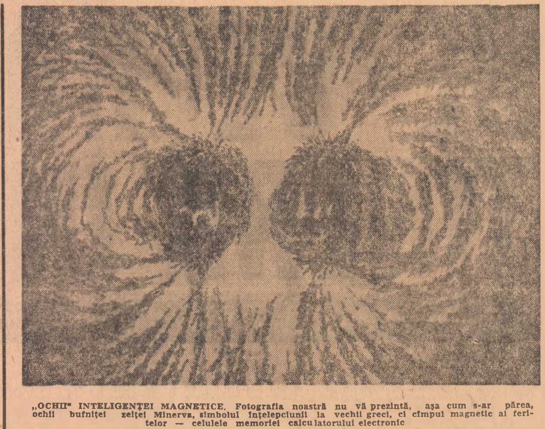
„OCHI” INTELIGENȚEI MAGNETICE. Fotografia noastră nu vă prezintă, așa cum s-ar părea, ochii bușniței zelei Minerva, simbolul intelctului la vechii greci, ci cîmpul magnetic al feritelor — celulele memoriei calculatorului electronic
