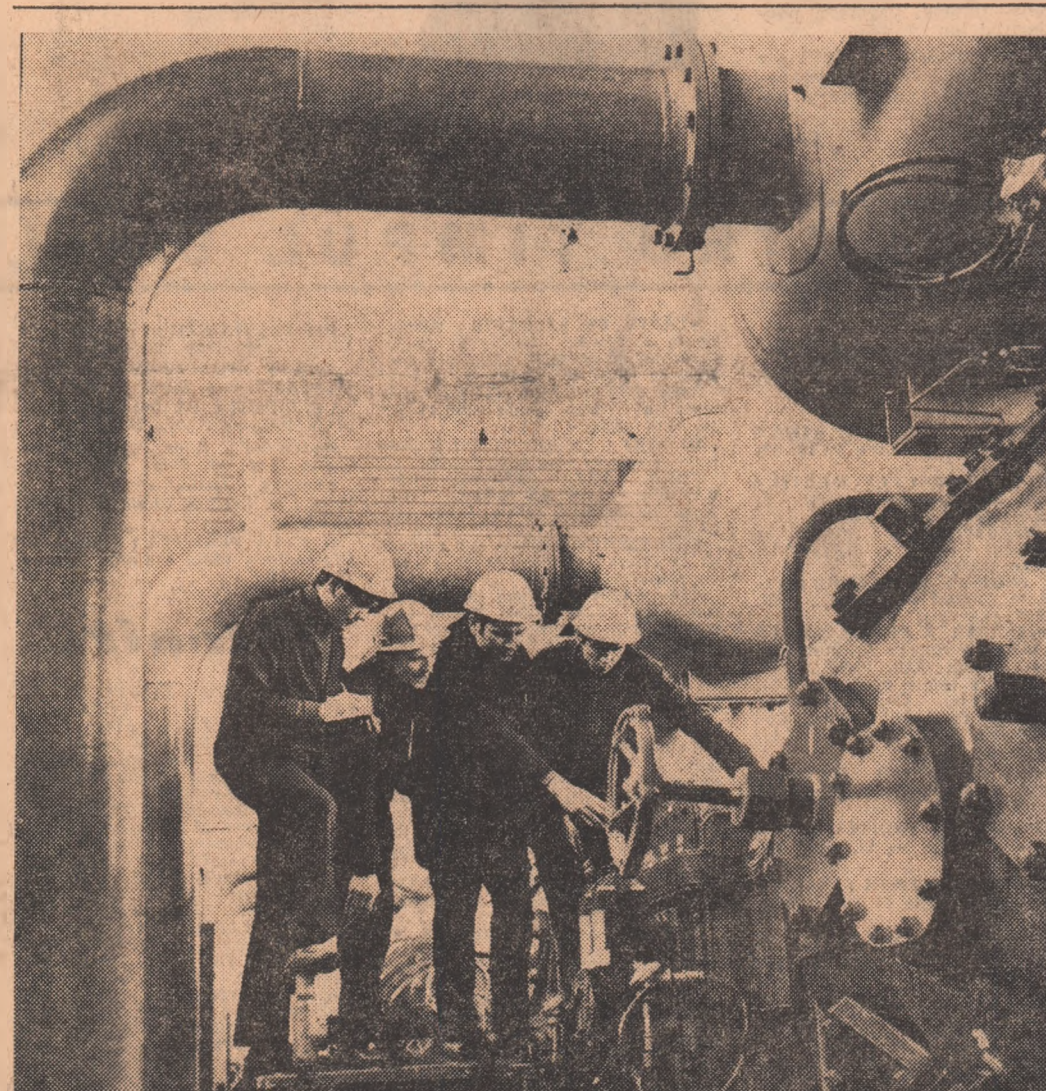
Combinatul chimic Craiova. Aflați în prezent în probe tehnologice, secția uree II, va intra în producție. Fotografia noastră îl înfățișează pe maestrul chimist Ion Rila, explicînd unui grup de tineri funcționarea utilajului la care vor lucra.
