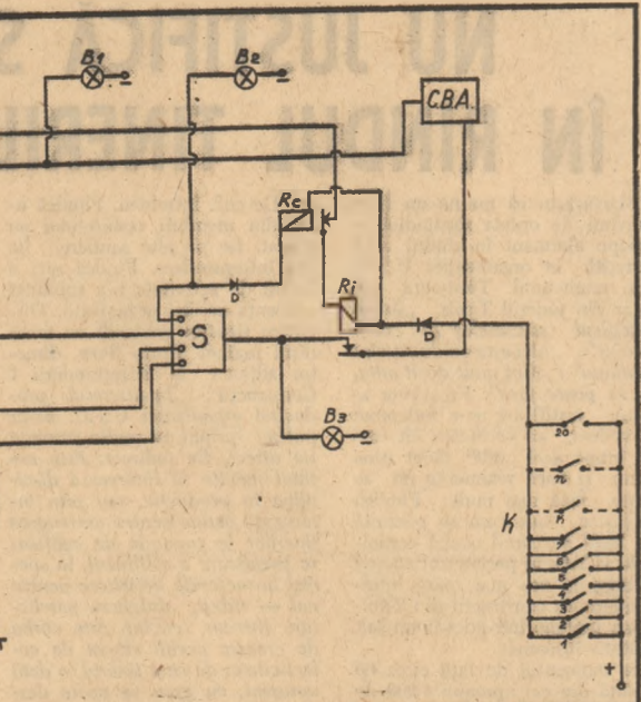
LEGENDA C.B.A. — Circuit basculant stabil; C.B.B. — Circuit basculant instabil; S — Selector; C.B. — Corp basculant; M — Monedă; B — Semnal luminos, anunțînd începerea jocului; B- — Se repetă jocul, fără a introduce monedă; B+ — Ciștiș; K — Blocul celor douăzeci de contacte.
