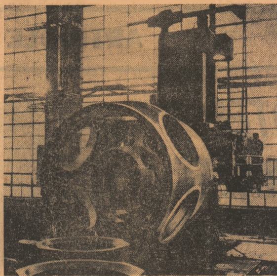
Reșița, secția mecanică grea. Aici se lucrează butucul rotorului turbinei de 176 M W. pentru Porțile de Fier.
