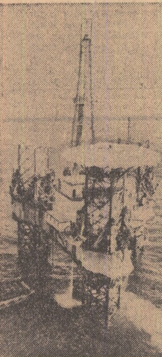
REPUBLICA MALGAȘĂ. — Platformă de prospecțiuni submarine, efectuînd cercetări în largul mării.
