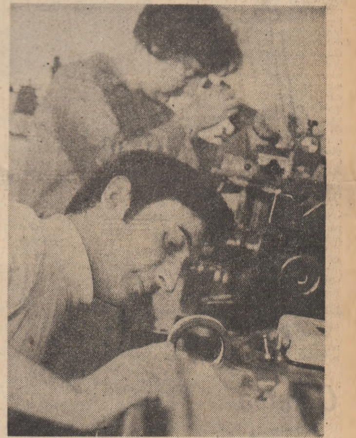
Uzina "Rulmentul" din Brayov. In imagine Bancila Ion si Sitarus Alexandrina - doi dintre muncitorii fruntasi ai intreprinderii - efectueaza controlul etaloanelor pe optometre
