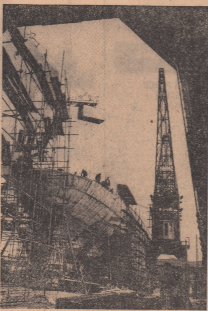
Șantierul naval Turnu Severin. Cargoul de 2000 tone capătă contur. Foto: O. PLECAN
