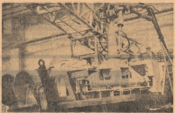
CPL 20 — o mașină care își sapă groapa dar nu cade în ea deoarece are un dispozitiv cu care o umple la loc.
