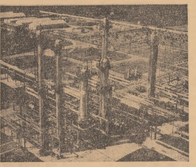
În imagine, uzina de gaz natural de la Hajdúszoboszóló, prin ale cărei conducte, 4 milioane de metri cubi de gaz ajung în fiecare zi în toate colțurile țării
