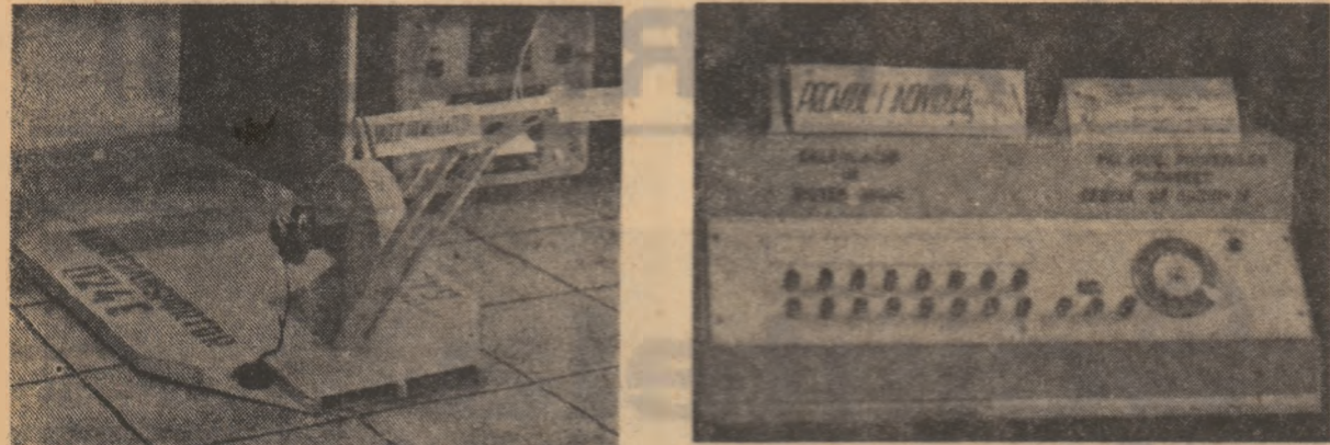
1. Aerotransportorul realizat de un colectiv de elevi din Galați, sub îndrumarea profesorilor Mihail Bănel, a obținut Marele premiu colectiv al expoziției. Funcționând pe principii pompei de aer, aparatul este capabil să transporte o greutate de 150 kg.
