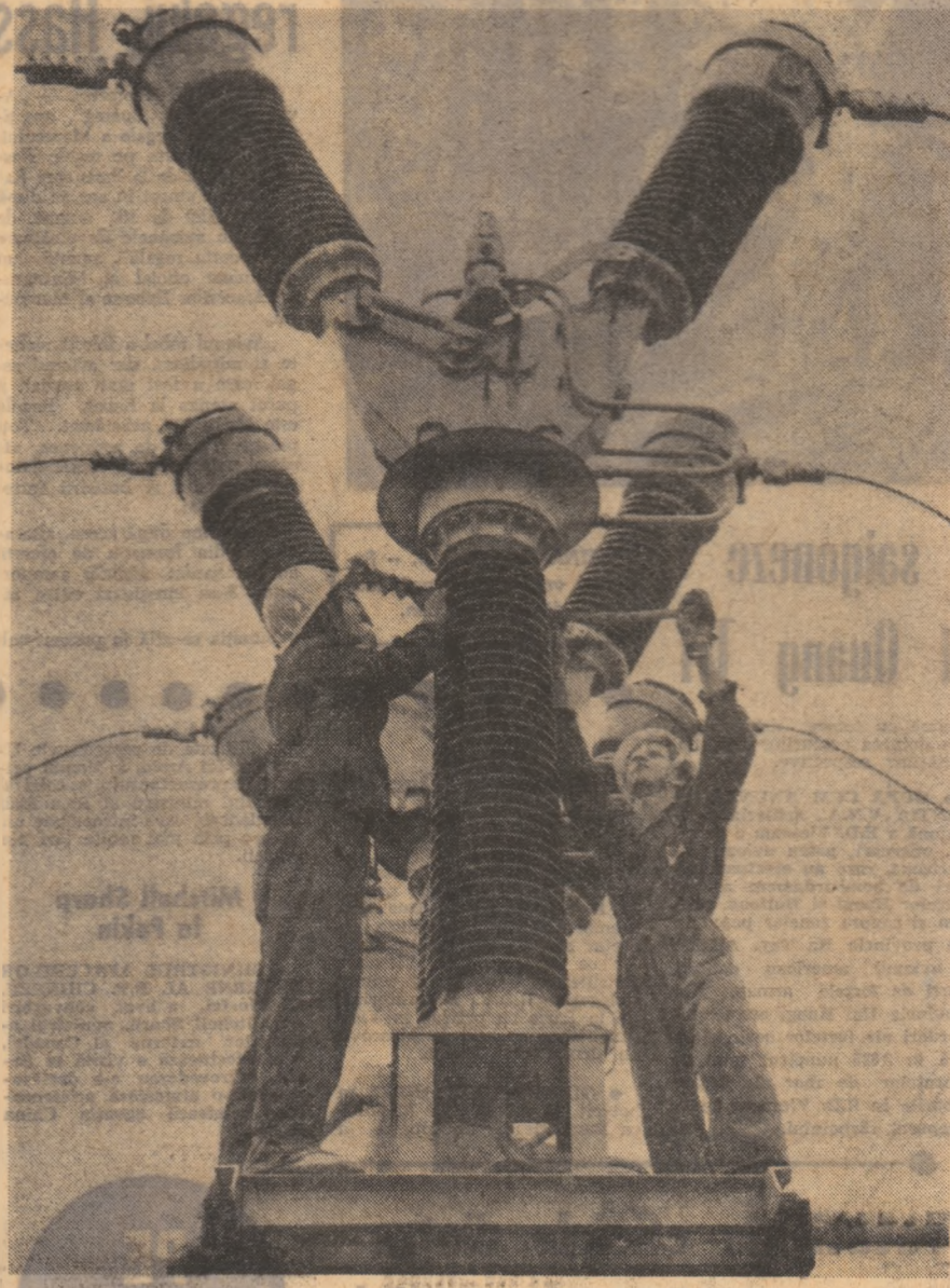
Se lucrează intens la un nou obiectiv industrial: stația de transformare a curentului electric ce va deservi Fabrica de piese de radio din Curtea de Argeș. În intensia constructorilor stă acum, darea în folosință cu șase luni înainte de termen.
