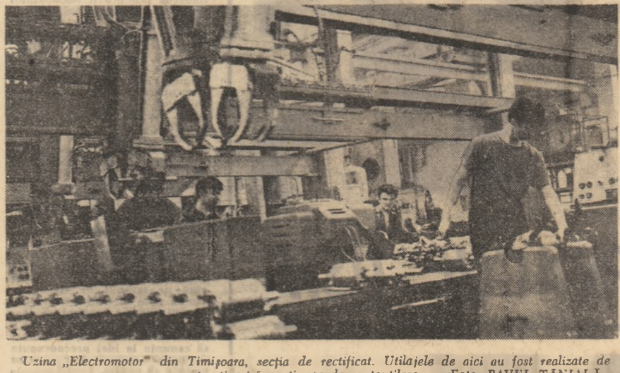
Uzina „Electromotor” din Timișoara, secția de rectificat. Utilajele de aici au fost realizate de către tineri în acțiunea de autoutilare. Foto: PAVEL TANJALA
