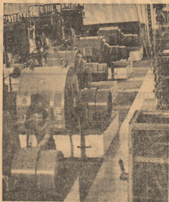
Sala compresoarelor a Exploatării miniere Herja. O unitate anexă esențială care acum un sfert de veac nu exista nici în cele mai frumoase cise ale ortacilor.
