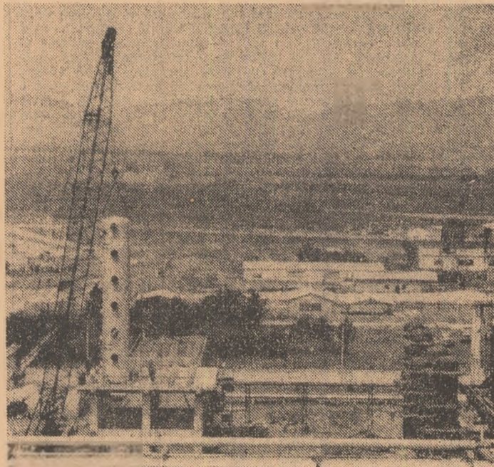
Combinatul petrochimic Borzesti. Vedere de ansamblu a lucrărilor de montaj ce se execută la stația de frig necesare capacității la Uzina de cauciuc sintetic.
