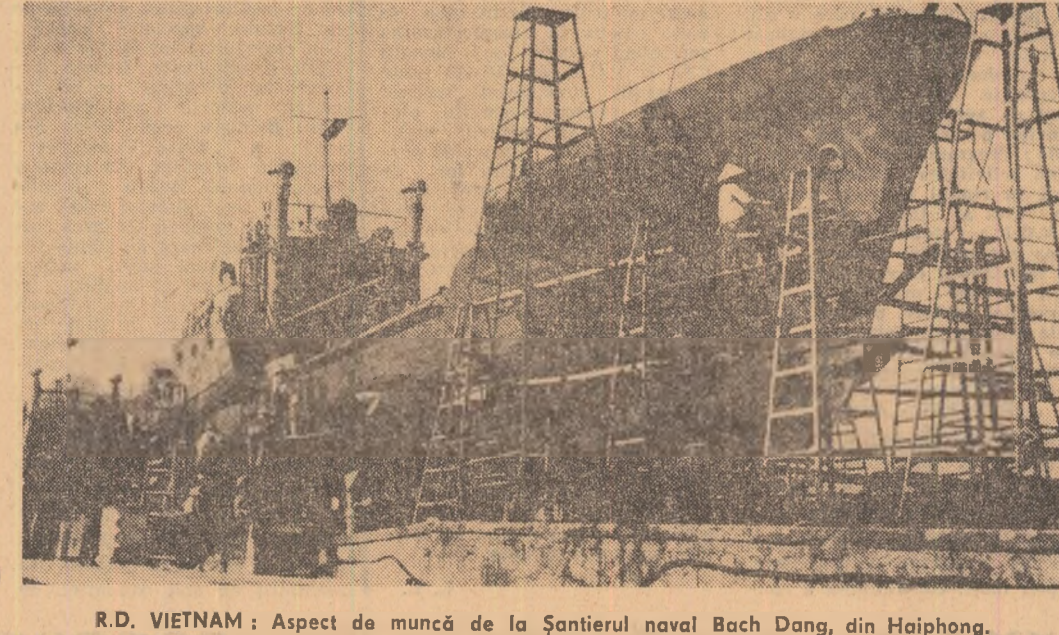
R.D. VIETNAM: Aspect de muncă de la Șantierul naval Bach Dang, din Hoiphona.
