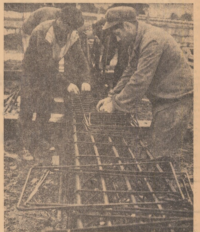
Se pregătește armătura metalică pentru hala de prefabricate a Fabricii de încălziminte „Progresul”.
