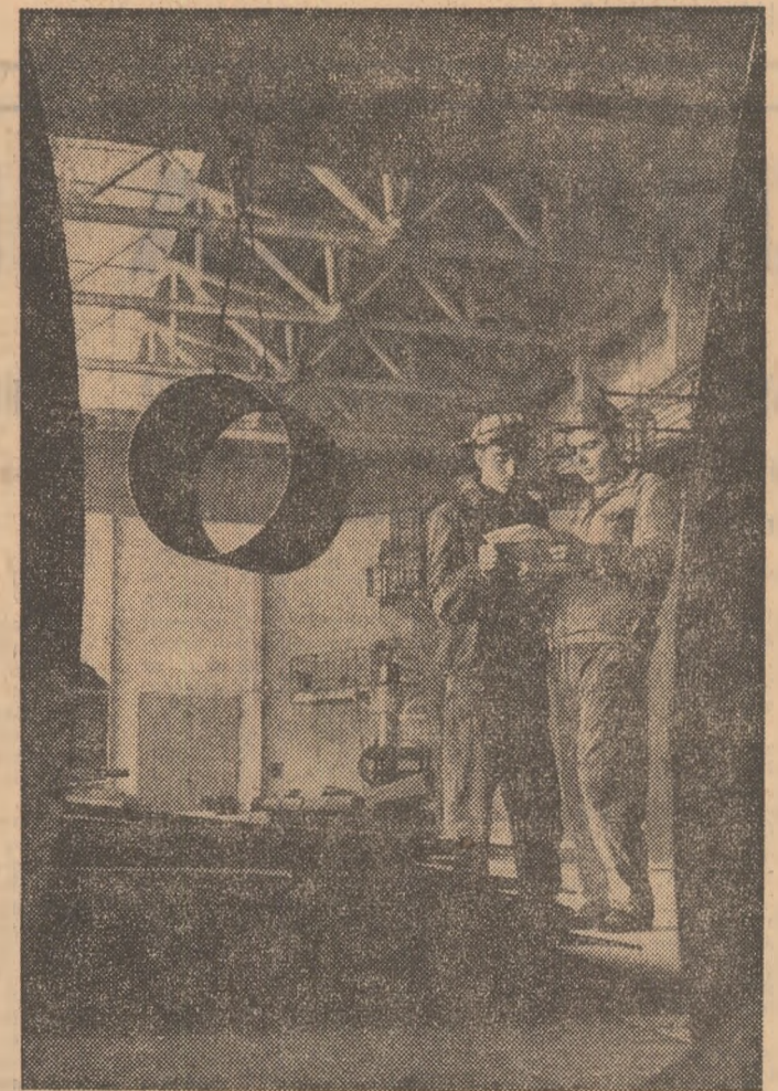
Economii de metal prin „croieli” ca la carte, respectînd la milimetru desenele tehnologice, iată numai unul din angajamentele asumate de tinerii cazanji, cu prilejul ultimei vizite făcute de conducătorul partidului și statului nostru la Întreprinderea de utilaj chimic din Căești. Un angajament care se înfăptuiește în fiecare zi
