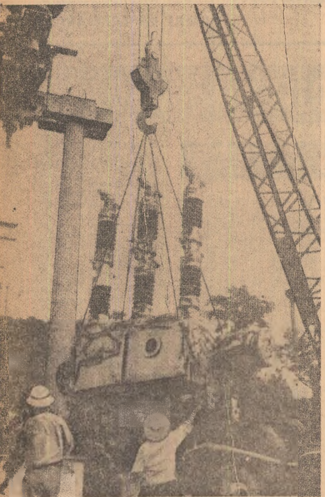
R. D. VIETNAM: lucrări la rețeaua de transformatori a hidrocentralei Thac Ba
