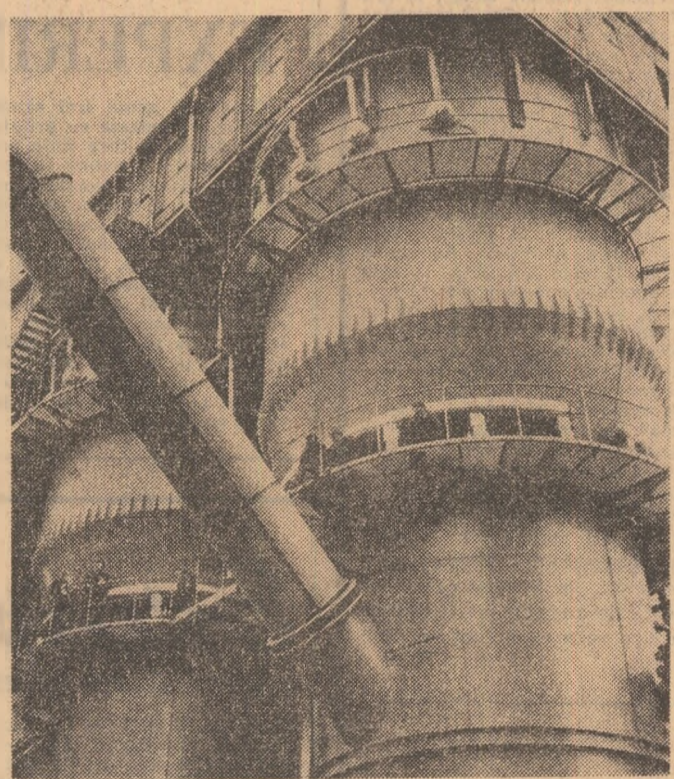
R.P. UNGARA. — Montajul unei instalații de purificare a aerului la Fabrica de aliaje din Zagyvarna.
