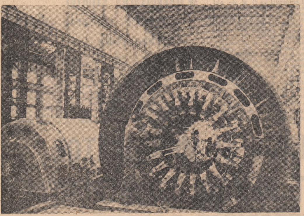
R.P. CHINEZĂ: Montarea unui turbogenerator de 125 MW la Uzina de mașini electrice din Șanhai
