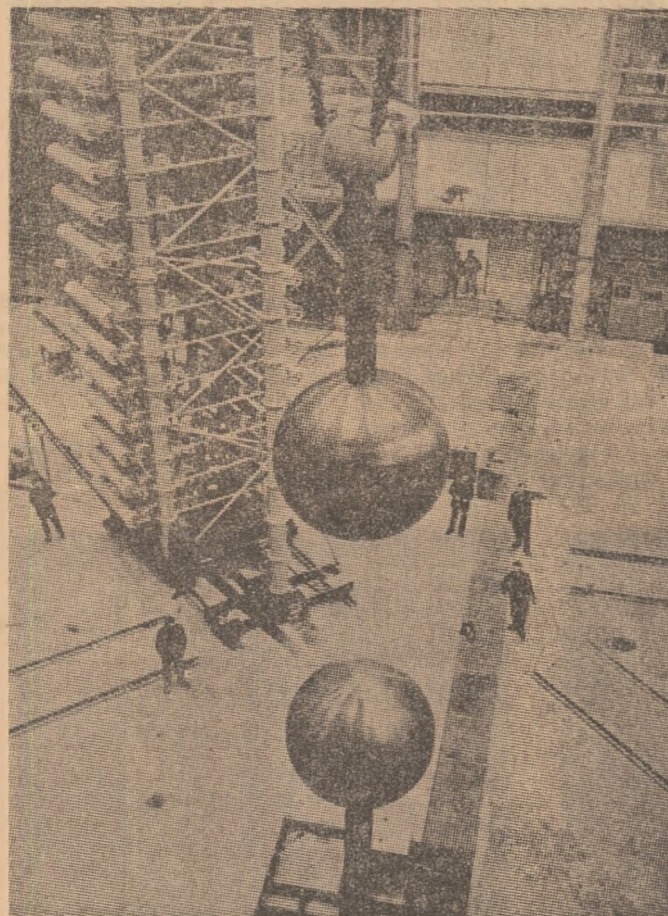
La Novosibirsk s-a construit o instalație unică în felul ei — un poligon de probe pentru curentul de înaltă tensiune. Aici oamenii de știință și inginerii de la Institutul de cercetări energetice din Siberia studiază procesele care se produc pe linia de înaltă tensiune.
