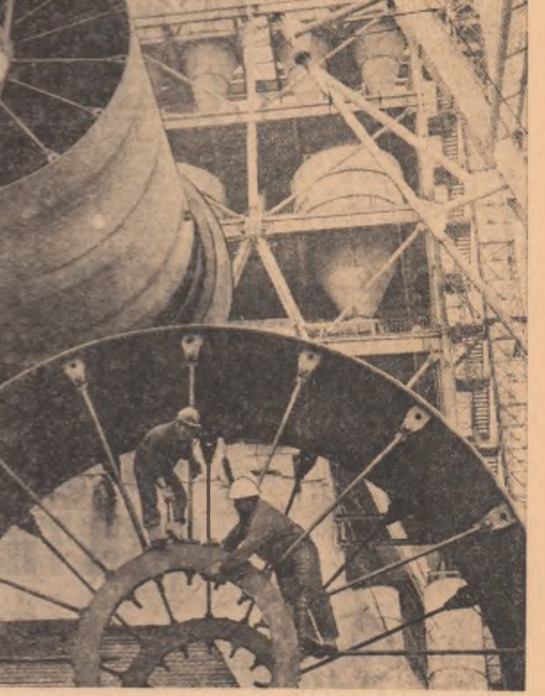
Fabrica de ciment și var, șantiernul 7 Deva, Chișcădaga. Aspect de la montarea cupturilor rotative nr. 1 cu o capacitate de 3000 t klingher pe zi. Foto: O. PLECAN
