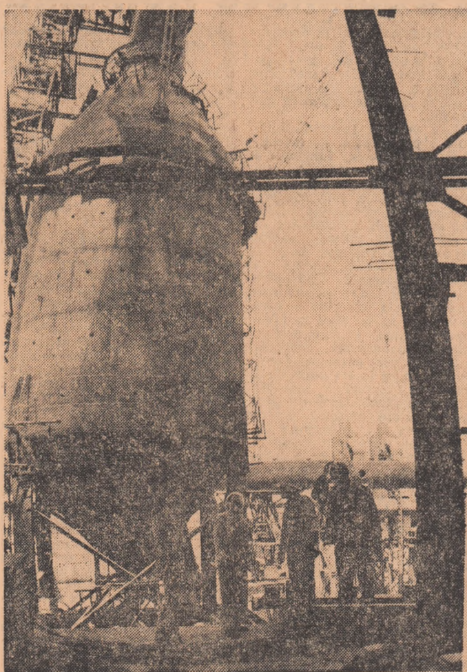
R. A. EGIPȚ: Aspect din timpul lucrărilor de construcție la cel de al patrulea furnal al Combinatului metalurgic din Helwan
