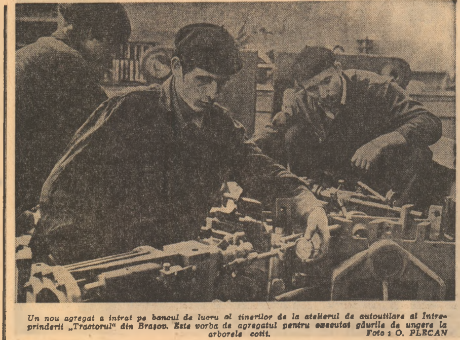
Un nou agregat a intrat pe bancul de lucru al tinerilor de la atelierul de autoutilare al întreprinderii „Tractorul” din Brașov. Este vorba de agregatul pentru evacuarea așterii la arborele cotit. Foto: O. PLECAN
