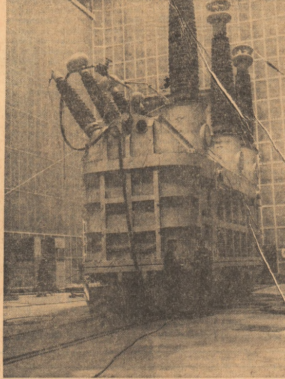
Aspect din laboratorul de înaltă tensiune al întreprinderii Electroputere-Craiova
