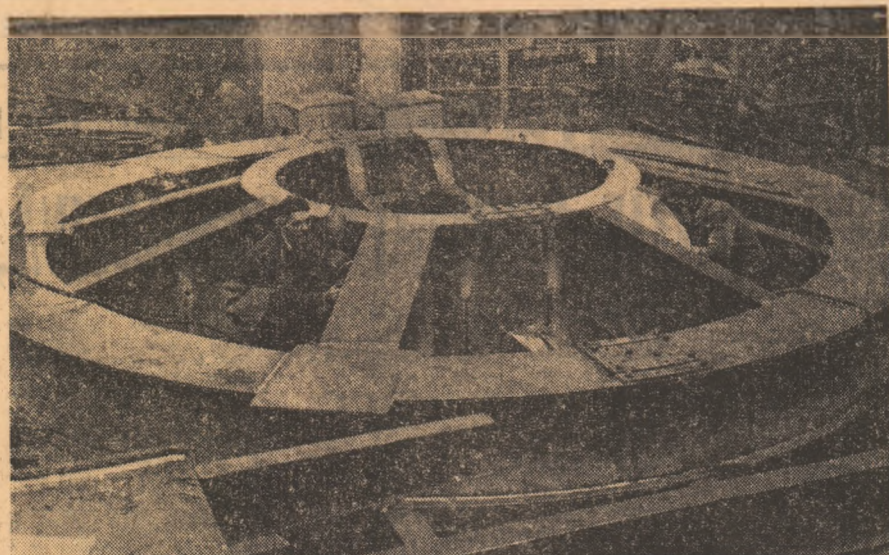
UZINELE MECANICE TIMIȘOARA. În execuție unul dintre cele mai importante repere pentru podurile rulante de turnare.
