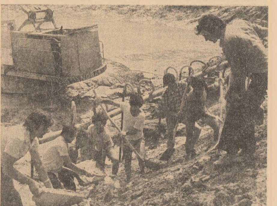
Șantierul sistemului de irigații Nedeia-Măceșu: Pe aici vor trece apele pentru rodnicia ogoarelor
