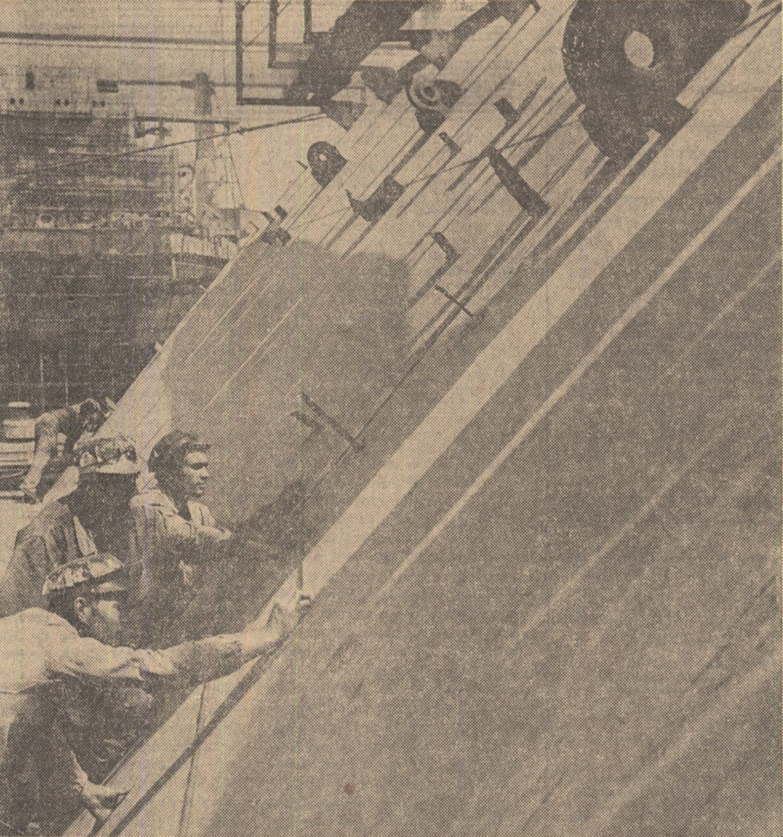
SANȚIERUL NAVAL CONSTANȚA. Deși uriasă, subansamblele trebuie sudate și montate cu precizie, operație pe care o verifică Costea Tănase, Părdălescu, Alexandru, Balanțu Teofil, de la atelierul montaj blocuri, secția I navală
