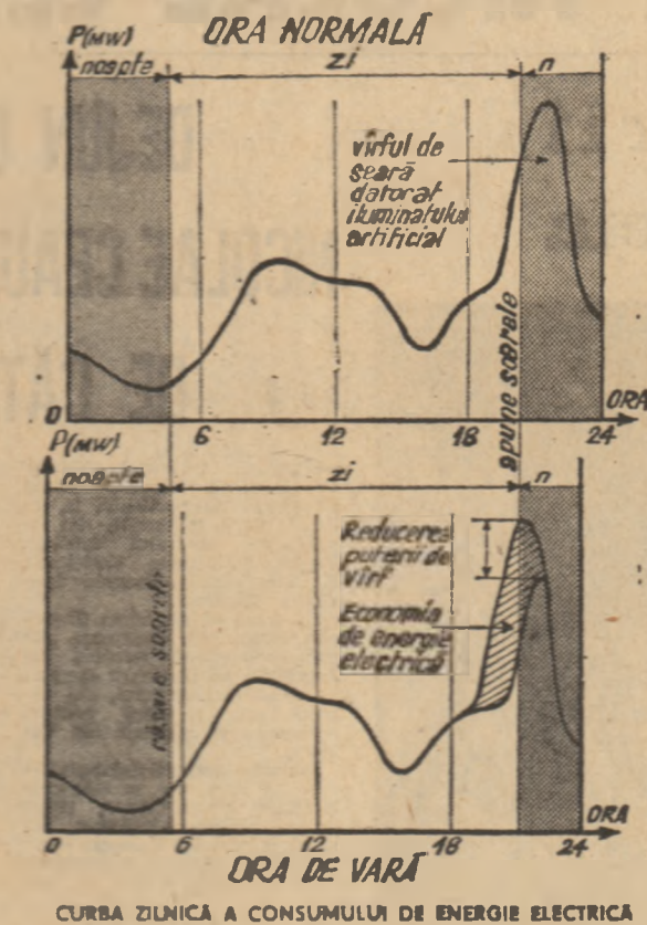
CURBA ZILNICA A CONSUMULUI DE ENERGIE ELECTRICA
