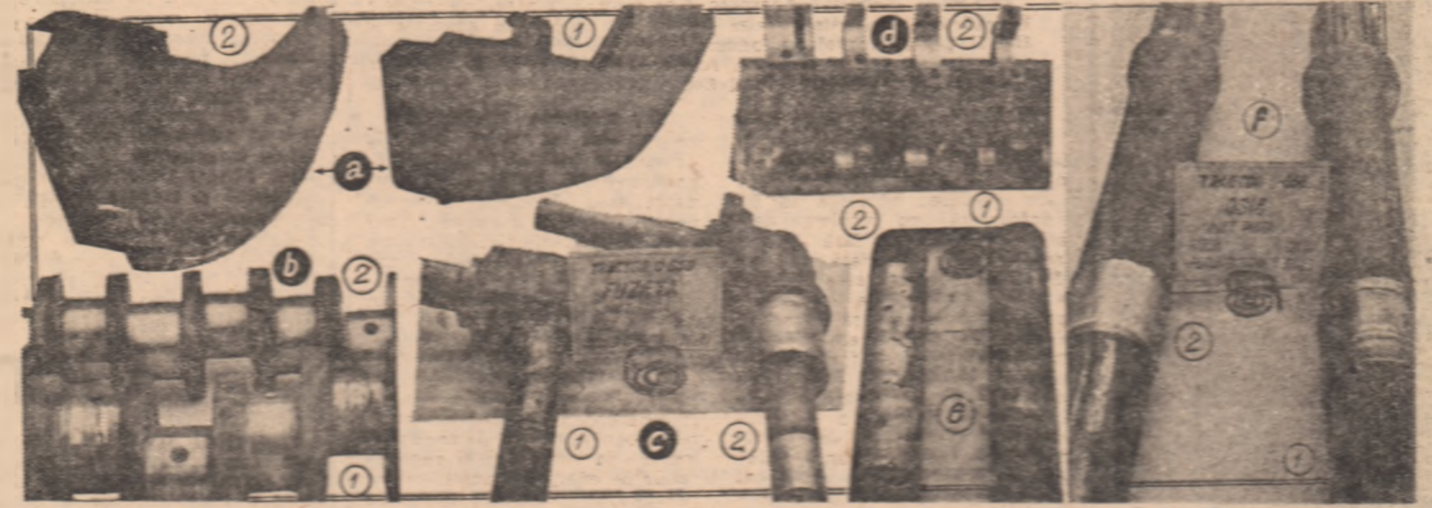
Fotomontaj prezintă multitudinea de posibilități pentru reintroducerea în circuitul productiv a pieselor de tractor și mașini agricole uzate, prin recondiționare: a) — potane semăntoare, b) — arbore cotit, c) — furcă, d) — bloc motor, e) — bare suport și direcție, f) — osie tractor. Rezerbuor, procedeu tehnic însoțind ados de material, supas apoi prelucrarea de fmețe micrometric sau milimetric în punctele de sprijin și elementelor în mișcare sau efort mecanic (1 — înainte de recondiționare, 2 — după recondiționare).
