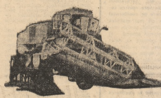
Deținătoare a mai multor diplome și medali de aur: combinația tractorului CP-12 pentru recoltat pășuni în pantă...
