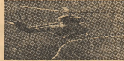
I.A.R.-330 Puma, elicopter reactiv mediu, viteza de croazieră 272 km/h, viteza maximă 281 km/h, plafon practic 4 600 m, încărcătură utilă 3 358 kg
