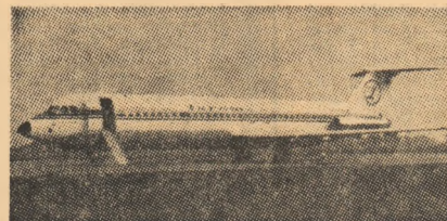
ROMBAC 1-11, aeronavă din clasa mediu-curier, cu viteza de croazieră de 870 km/h la altitudinea de 11 000 m, 110 sau 119 locuri, cu o autonomie de zbor de peste 3 000 km
